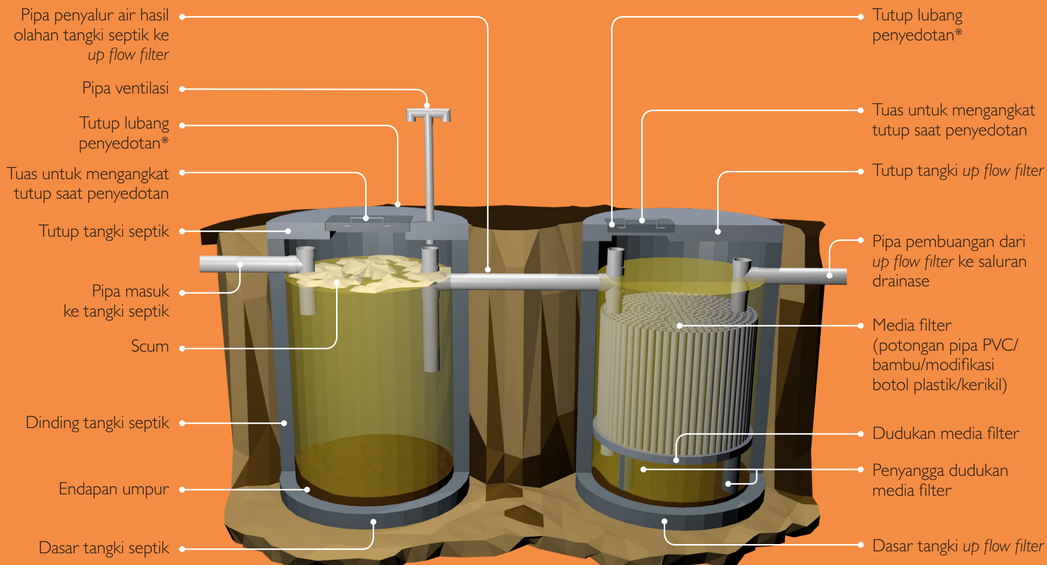
TANGKI SEPTIK
